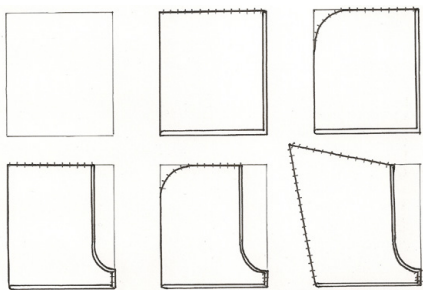
Abb. 99 | Konstruktions-, Schnitt- und Nahtlinien
