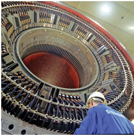
Abb. 156 | Riesiger Generator der Firma Siemens
