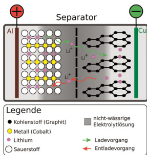
Abb. 118 | Funktionsprinzip eines LI-Akkus. Die LI-Ionen verschieben sich beim Laden und Entladen zwischen den beiden Elektroden.
