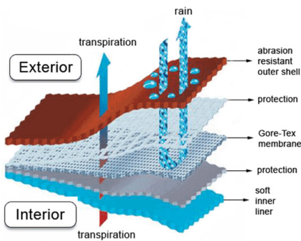
Abb. 77 | Aufbau von Goretex Textilien
