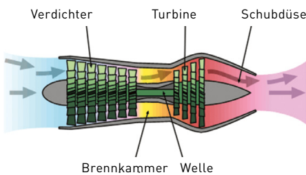
Abb. 275 | Prinzip des Strahltriebwerks
