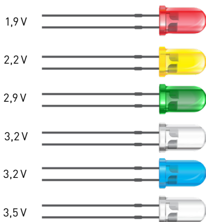
Abb. 158 | Durchlassspannung verschiedener LEDs
