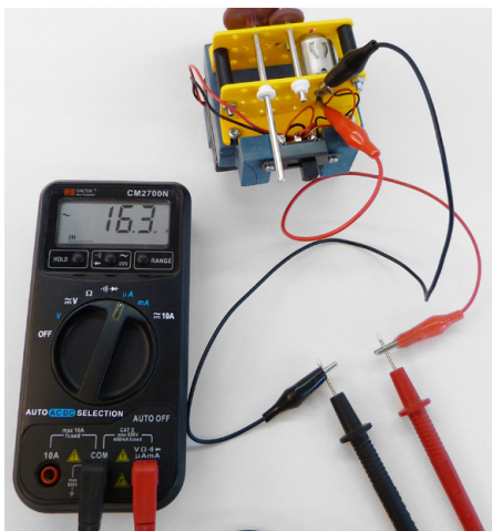
Abb. 160 | Strommessung an einem Getriebemotor
