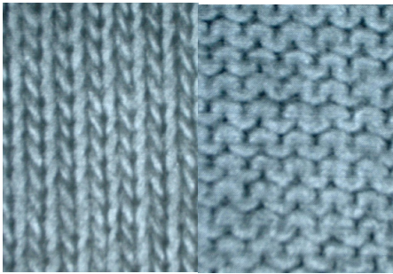
Abb. 90 | Rechte und linke Wareseite einer RL-Bindung (auch Single Jersey)
