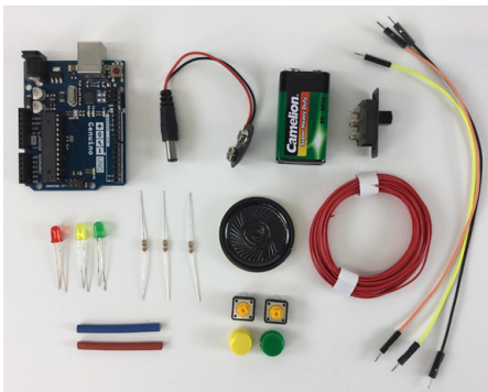
Abb. 193 | v. l. n. r.: Arduino UNO, Batterie-Clip, 9V-Batterie, Schalter, Jumperkabel, LED, Widerstand, Lautsprecher, Schalt- oder Litzendraht, Schrumpfschlauch, Taster
