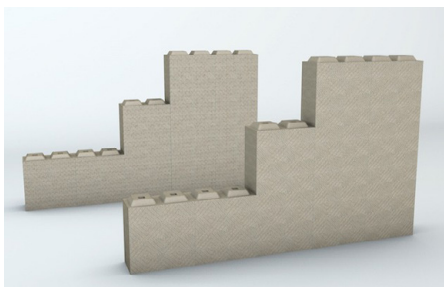
Abb. 318 | Alternative zum herkömmlichen Beton: Polymerbetonsteine, die sich stapeln lassen
