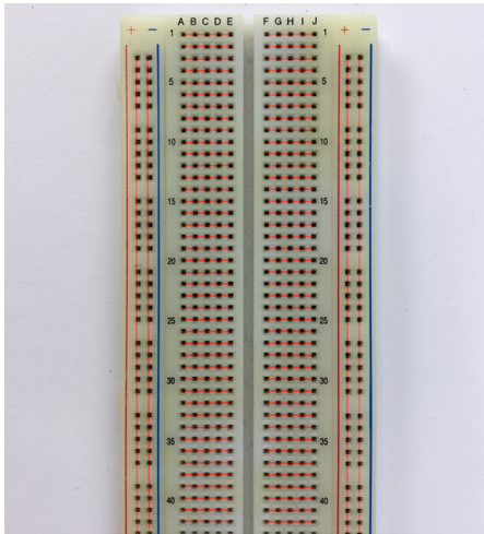
Abb. 192 | Steckplatine mit eingezeichneter Linie zum Stromfluss
