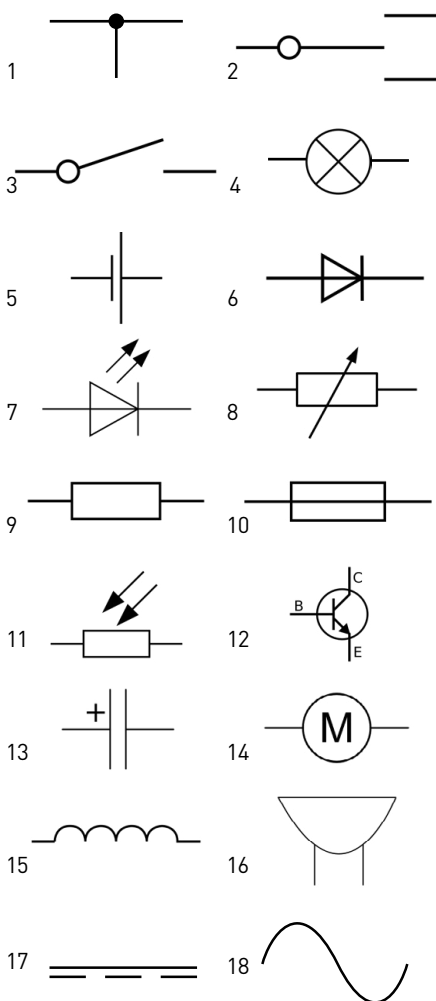
Abb. 157 | Schaltsymbole: 1: Leiter mit Verzweigung, 2: Umpolschalter, 3: Schalter, 4: Glühlampe, 5: Batterie, 6: Diode, 7: Leuchtdiode (LED), 8: Potenziometer, 9: Widerstand, 10: Sicherung, 11: Fotowiderstand, 12: Transistor, 13: Elko (gepolter Kondensator), 14: Motor, 15: Spule, 16: Summer, 17: Gleichstrom, 18: Wechselstrom
