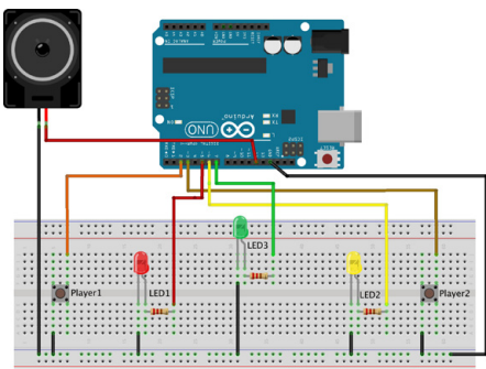
Abb. 191 | Schaltplan von «Ready-Steady-Baam» in der Steckplattenansicht
