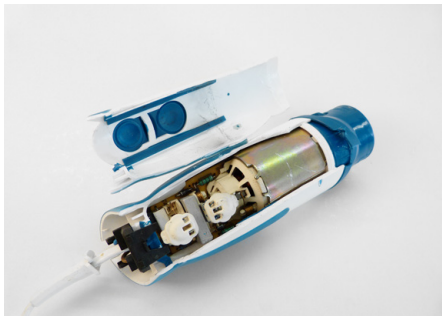
Abb. 155 | Elektromotor eines Küchenmixers
