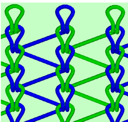
Abb. 93 | Schema der Trikotlegung
