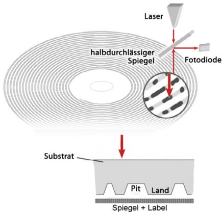
Abb. 177 | Auslesevorgang bei einer CD. Das Licht trifft auf die Pits und Lands und wird entsprechend reflektiert.
