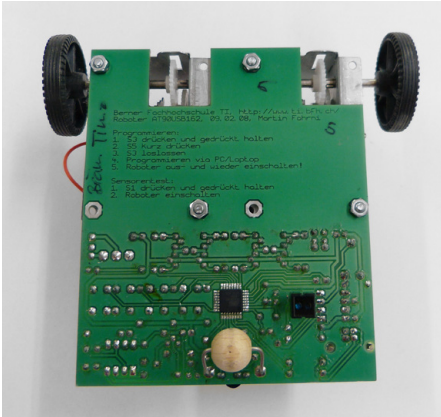
Abb. 184 | Der Microcontroller als Gehirn eines Roboters
