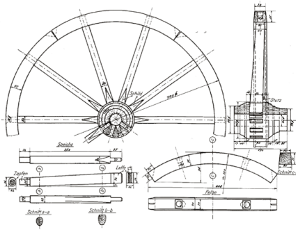
Abb. 269 | Sturzrad: Skizze eines eisenbereiften Sturzrads mit Holznahe
