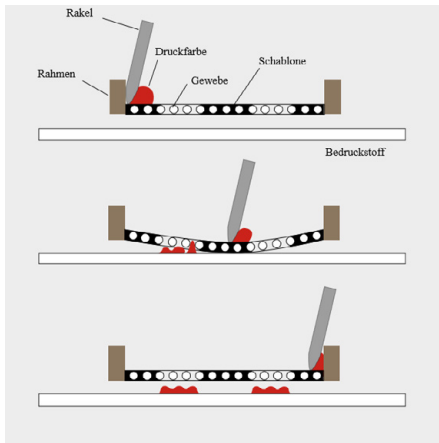
Abb. 99 | Schema des Siebdruckverfahrens
